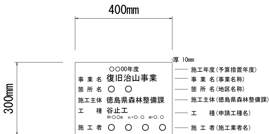
図1 銘板の寸法及び記載事項
